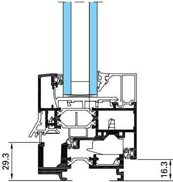
BALCONERA 2 HOJAS CON PERFIL SUELO PRM APERTURA INTERIOR
