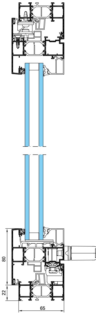
VENTANA ITALIANA APERTURA EXTERIOR
